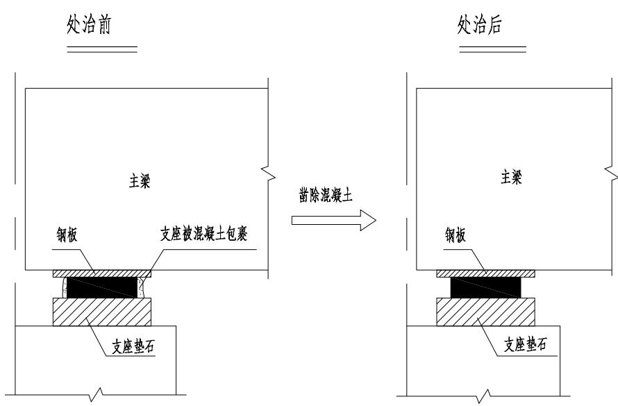
支座被混凝土包裹处治示意
