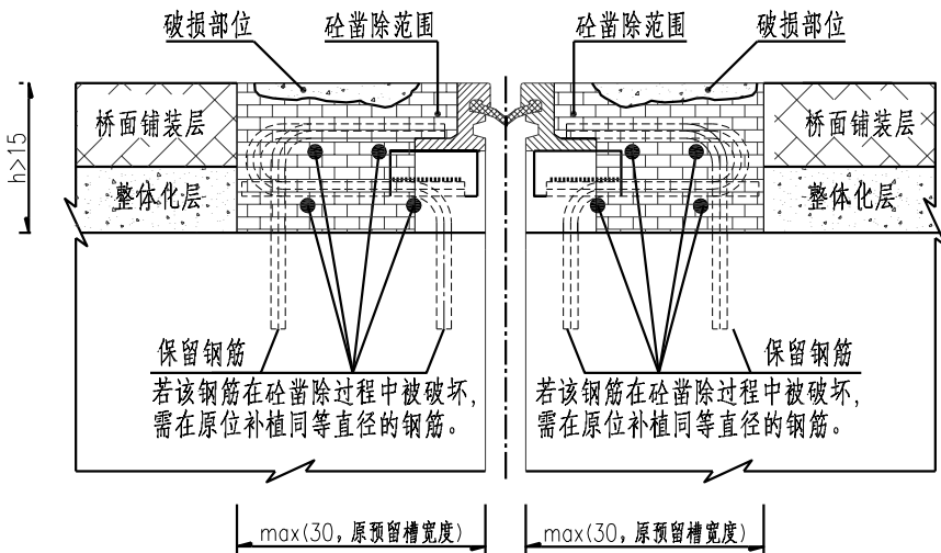
I—I (D80型伸缩缝)
