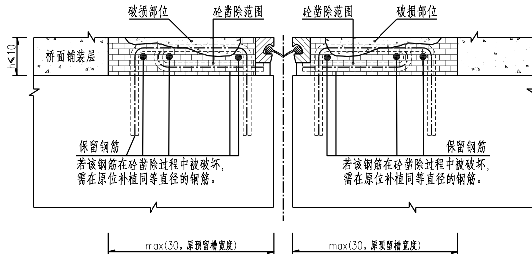
I—I (浅埋式伸缩装置)
