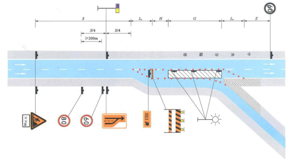
图 8-6 立交出口匝道附近封闭车道养护作业 (1)
